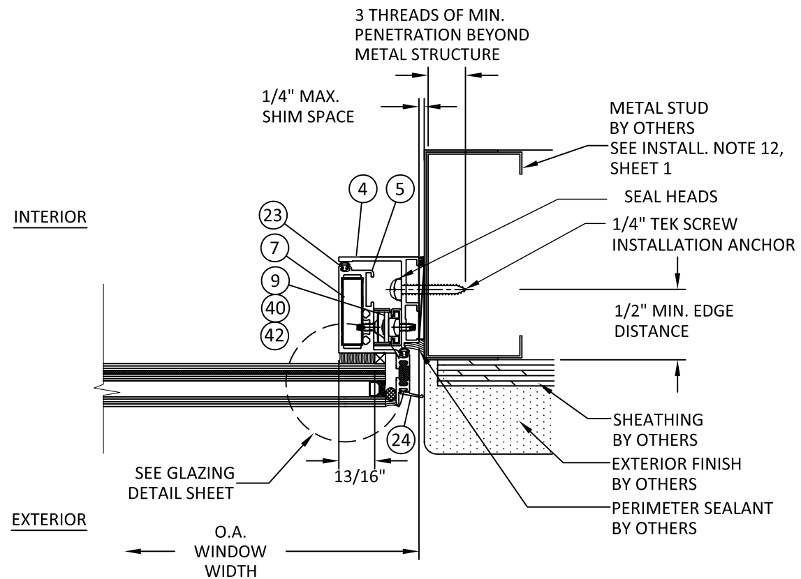
C 4 HORIZONTAL SECTION VENT JAMB - METAL STUD FRAME FLAT FRAME
